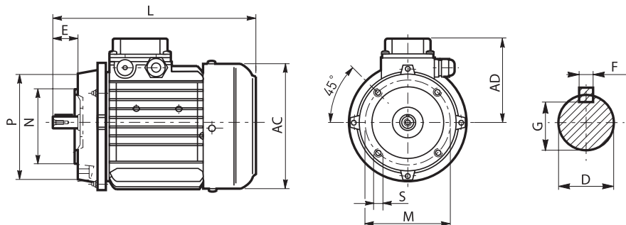
Исполнение IM B14
