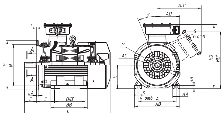
A-A исполнение 1
